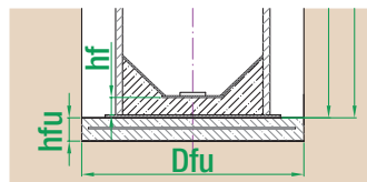
Stahlbetonfundament, Innen mit Betonfüllung
