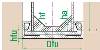
Stahlbetonfundament, mit Aufbeton, Innen mit Betonfüllung
