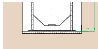
Sauberkeitsschicht Magerbeton
