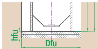
Stahlbetonfundament
